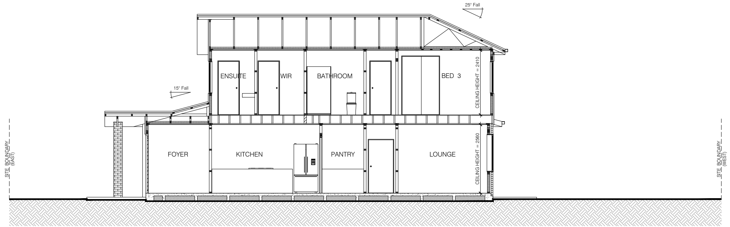
LONGITUDINAL SECTION
