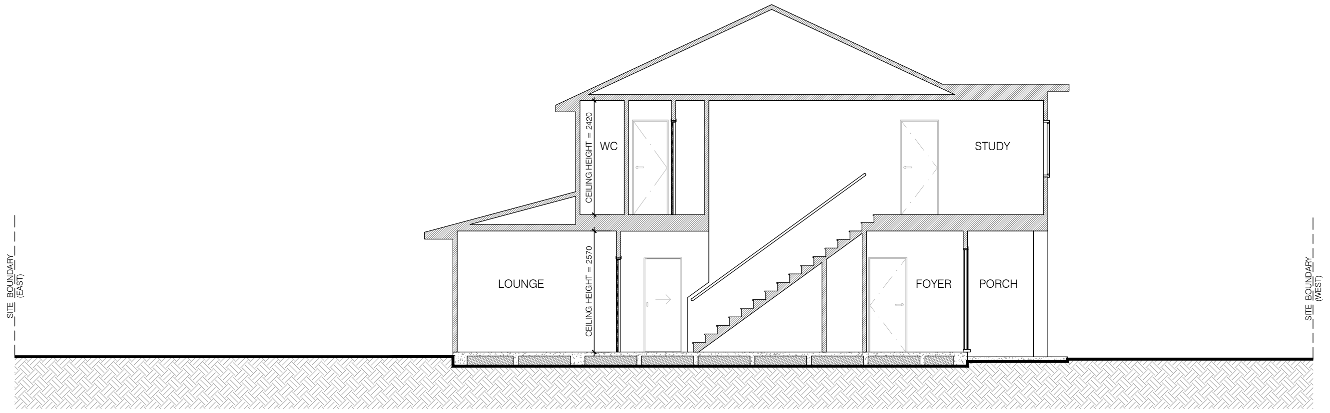
LONGITUDINAL SECTION
